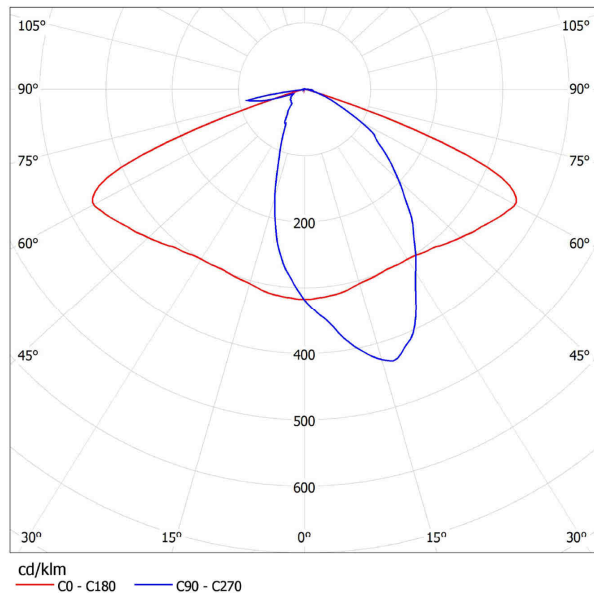
Courbe de distribution pour URSA II LED ALFA
