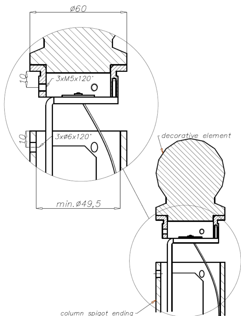
Plan de montage sur le mât pour un emmanchement de Ø60
